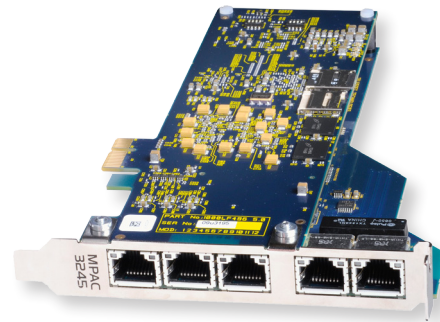
MPAC 3240 / 45 8 x E1 / T1 PCIe Card
